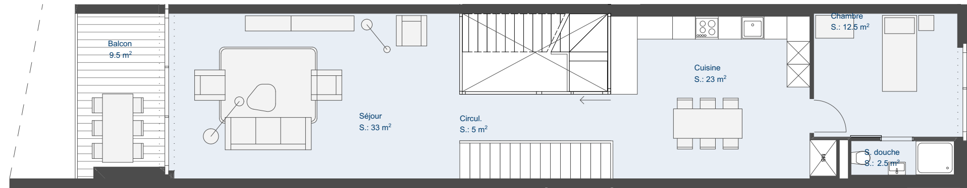
1er étage
